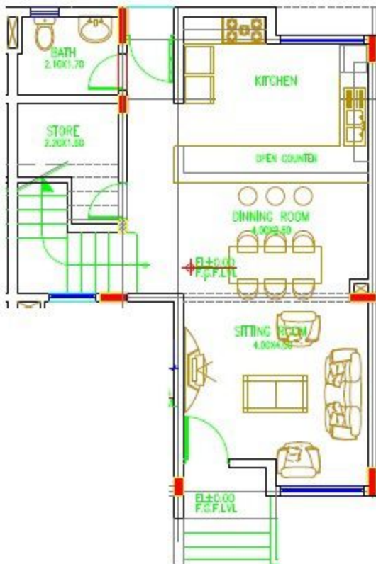
AJV1, 3BEDROOM VILLA GF
